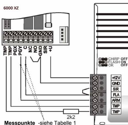
Abb. 3 Anschlussbeispiel mit der Zentrale 6000 XZ
