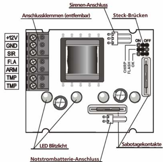
Abb. Oberseite der Platine
